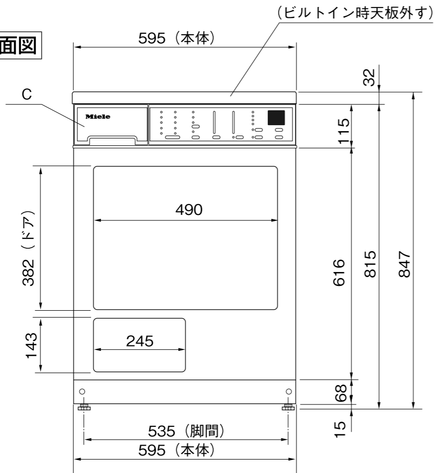
側面図
