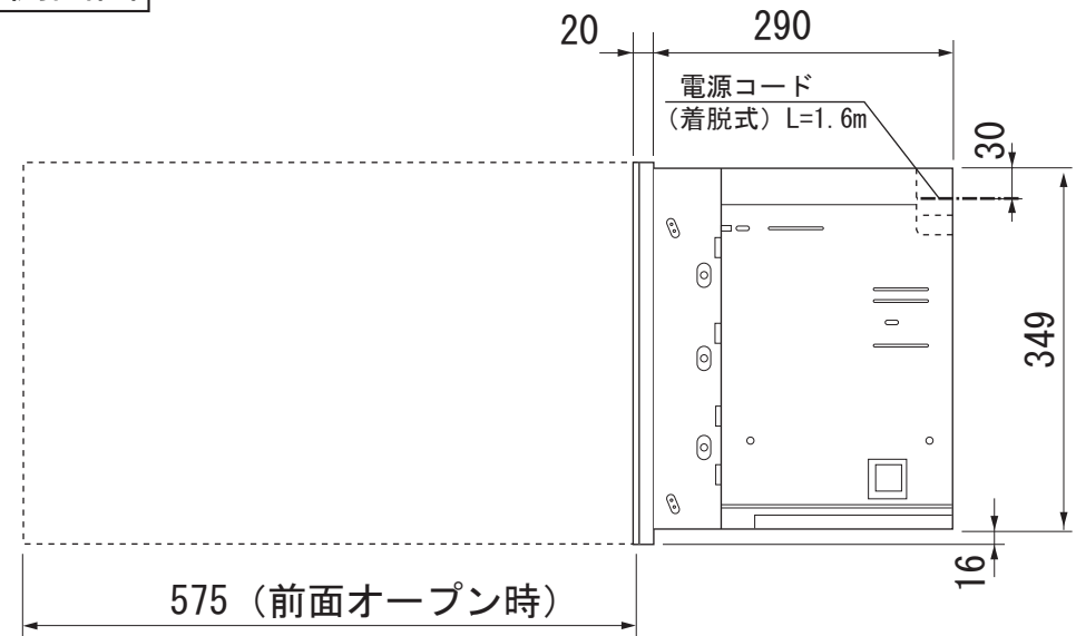
側面図
