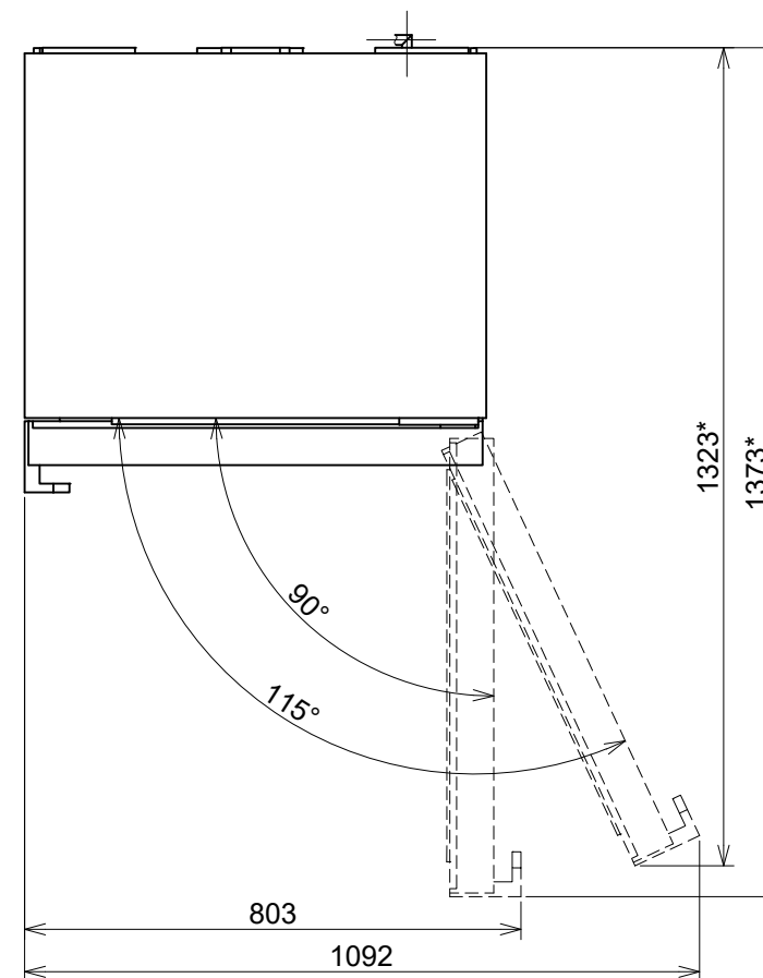
平面図
