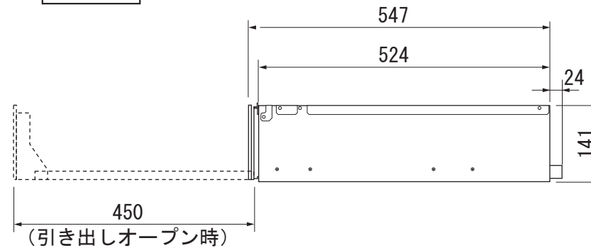
側面図
