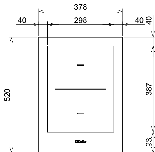
平面図
