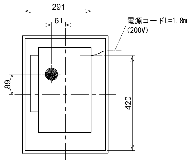
背面図
