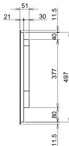
背面図
